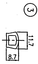
フッダ-カバー断面図 (S=1/1)
