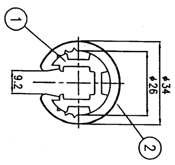
本体断面図 (S=1/1)
